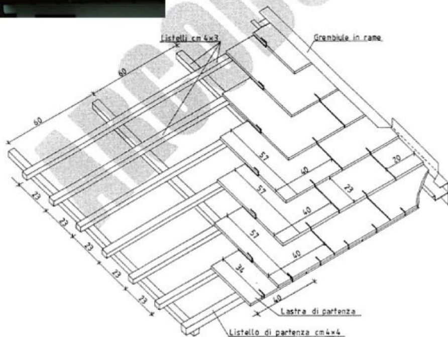
ASSONOMETRIA SCHEMATICA
