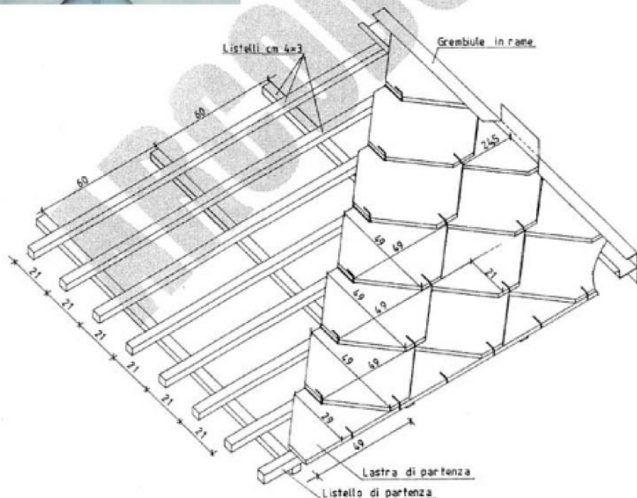
ASSONOMETRIA SCHEMATICA
