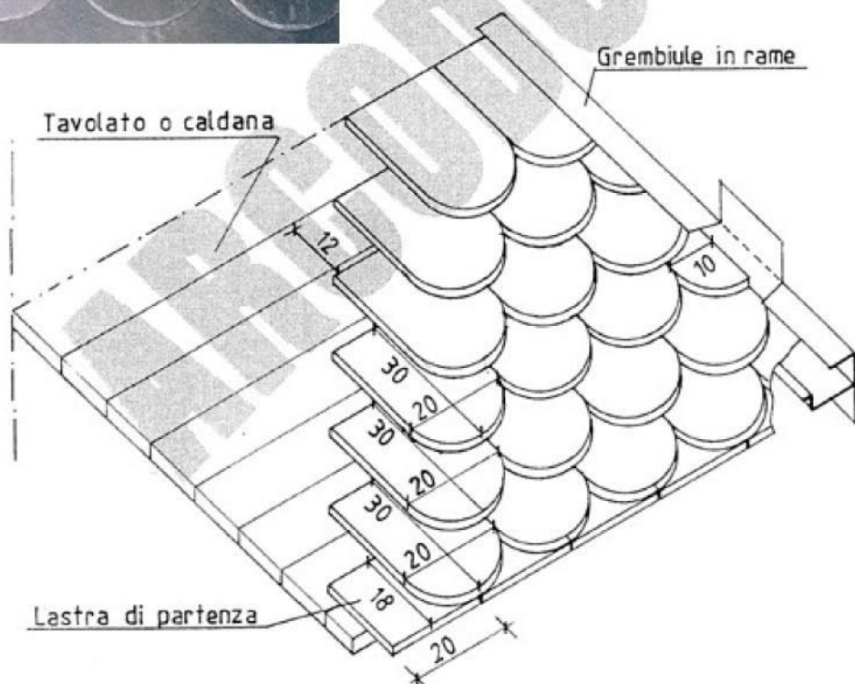
ASSONOMETRIA SCHEMATICA
