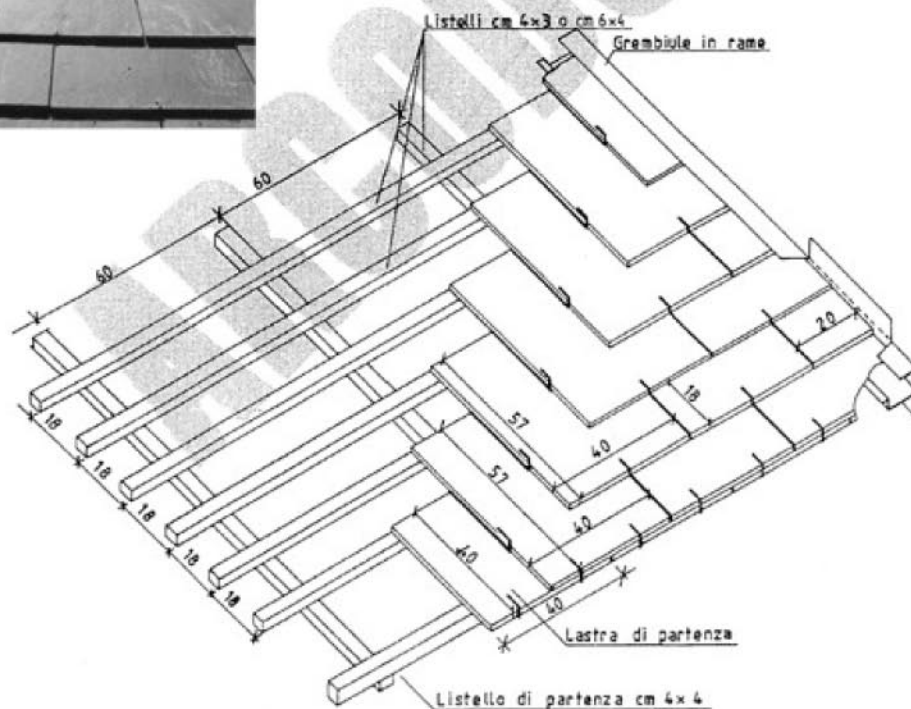
ASSONOMETRIA SCHEMATICA
